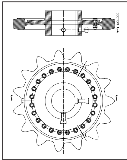
Segmental Sprocket
