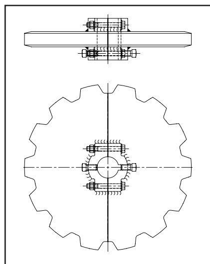
Split Sprocket
